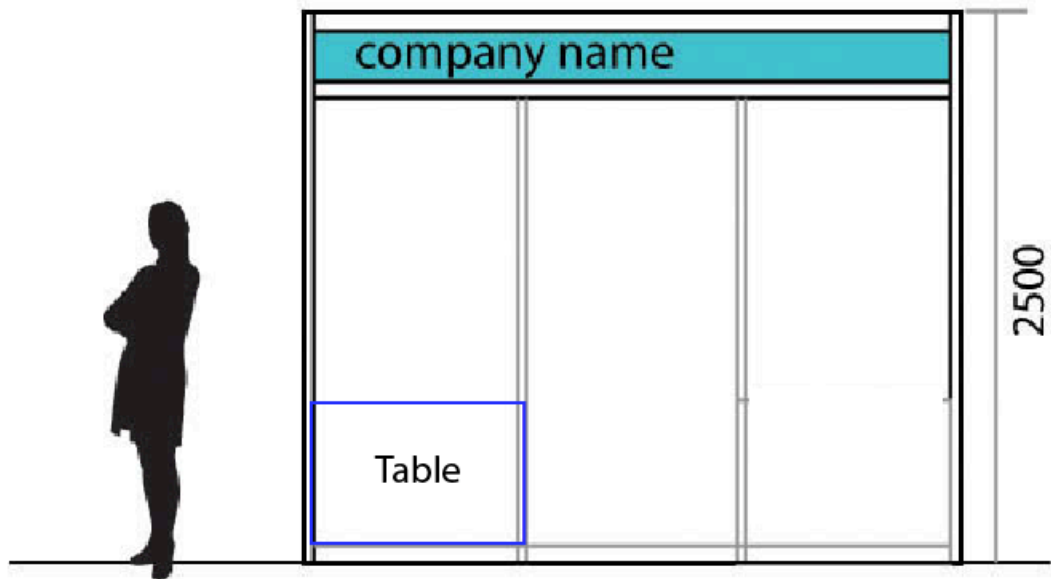
立面圖 A Front Elevation
