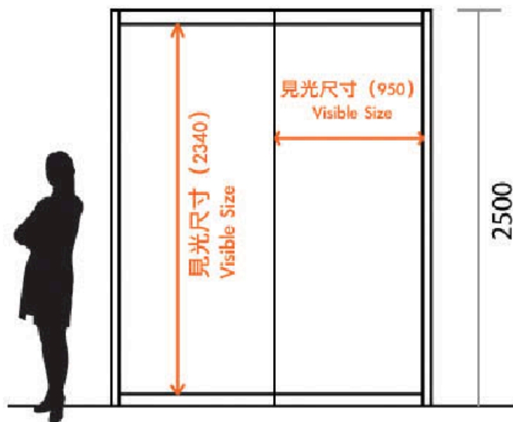
側面圖 B End Elevation
